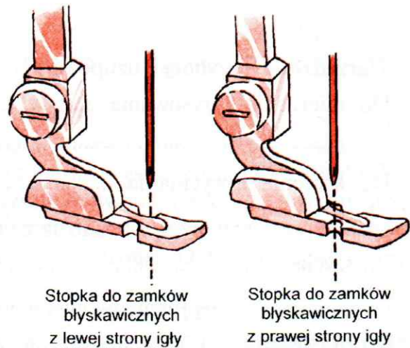
Rys. 7d. Stopki do zamków błyskawicznych
