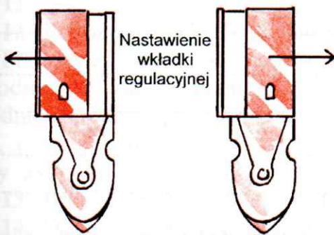
Rys. 7c. Wkładki regulacyjne
